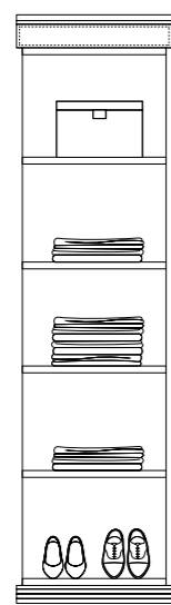
SN101 senza anta SNV101 anta vetro SNL101 anta legno CM 60 X 60 X 235,5 H
