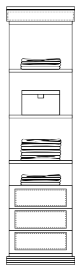
SN103 senza anta SNV103 anta vetro SNL103 anta legno CM 60 X 60 X 235,5 H
