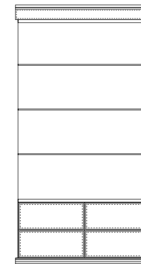
S006 senza anta SV006 anta vetro CM 120 X 46 X 235,5 H
