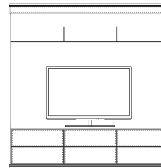
S009 senza anta CM 225 X 46 X 235,5 H
