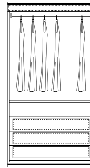
SN138 senza anta SNV138 anta vetro SNL138 anta legno CM 120 X 60 X 235,5 H
