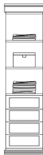
SN102 senza anta SNV102 anta vetro SNL102 anta legno CM 60 X 60 X 235,5 H
