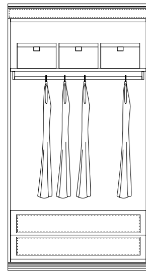
SN134 senza anta SNV134 anta vetro SNL134 anta legno CM 120 X 60 X 235,5 H
