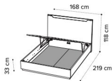
Letto SMART c/contenitore Luna e rete 160x200 SMART bed with Luna storage 160x200 Кровать SMART с полноразмерным мех-мом 160x200
