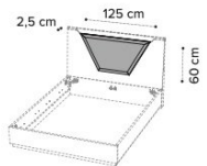
Cuscino testiera QS 154 letto SMART Cushion headboard QS 154 letto SMART
