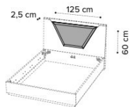
Cuscino testiera 160 letto SMART Cushion headboard 160 letto SMART
